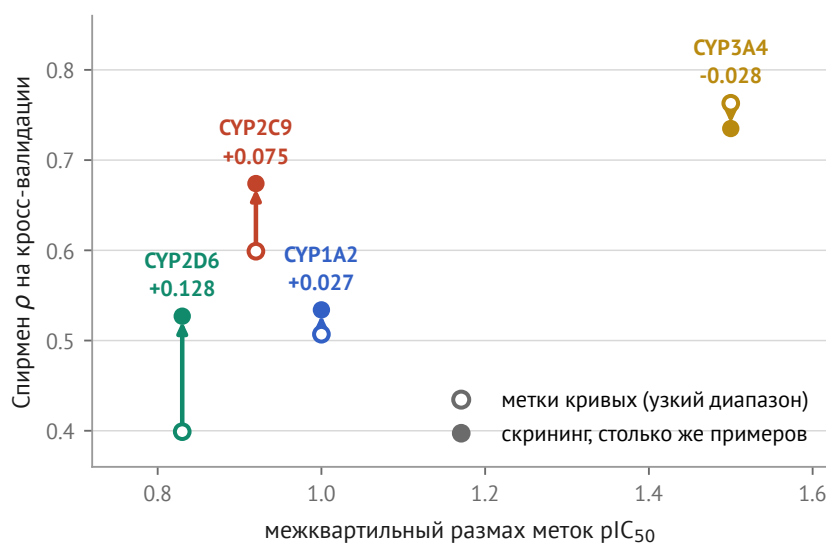
Рис. 3. Выигрыш от перехода на показатель с полным диапазоном против ширины полосы меток. Пустой кружок — качество на метках кривых, закрашенный — на скрининге при равном числе обучающих примеров. Стрелка тем длиннее, чем уже полоса меток, и на CYP3A4 разворачивается.
