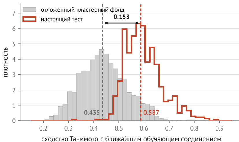
Рис. 9. Насколько далеко проверяемое соединение от того, что модель видела. Разрыв медиан 0.153, и он идёт в неожиданную сторону: наша проверка труднее теста. Эти две медианы взяты против опор разного размера — отложенное соединение сравнивается с четырьмя выборками, тестовое со всей, а максимум по большей опоре больше даром. Размерно сопоставленный разрыв даёт следующая таблица: 0.137 против leave-one-out, и он же выходит 0.131, если считать тест против случайных четырёх пятых. Вывод от этого не меняется, но пару чисел надо брать из таблицы, а не отсюда.
